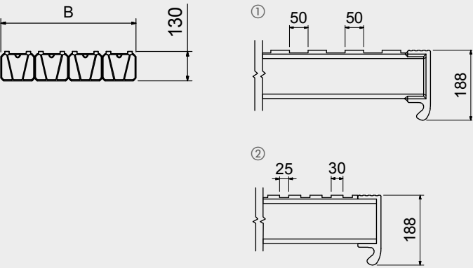
① EMPATTEMENT 50/50 (STANDARD) ② EMPATTEMENT SPÉCIAL 25/30 (SUR DEMANDE)
