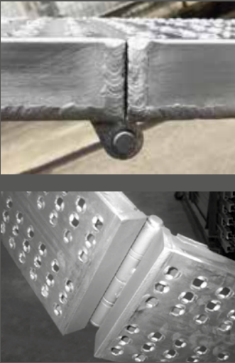
MODÈLE B2 À CHARNIÈRES (SUR DEMANDE)
