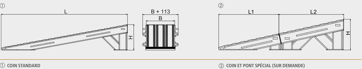
① COIN STANDARD ② COIN ET PONT SPÉCIAL (SUR DEMANDE)
