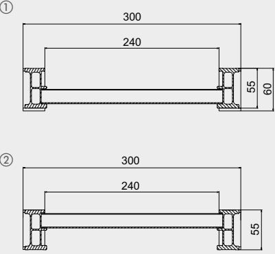
① AVEC BORDS ② SANS BORDS
