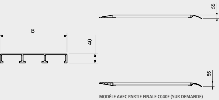
MODÈLE AVEC PARTIE FINALE C040F (SUR DEMANDE)
