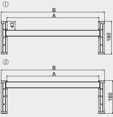
1 AVEC BORDS 2 SANS BORDS
