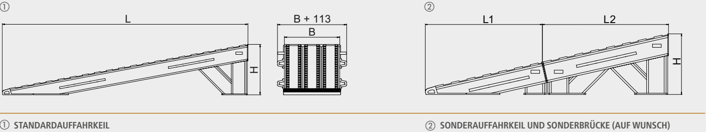
1 STANDARDAUFFAHRKEIL 2 SONDERAUFFAHRKEIL UND SONDERBRÜCKE (AUF WUNSCH)
