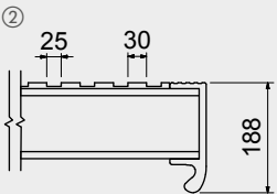
1 ABSTAND 50/50 (STANDARD) 2 SPEZIALABSTAND 25/30 (AUF WUNSCH)
