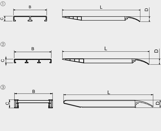
1 MODELL B2 2 MODELL B3 3 MODELL M065
