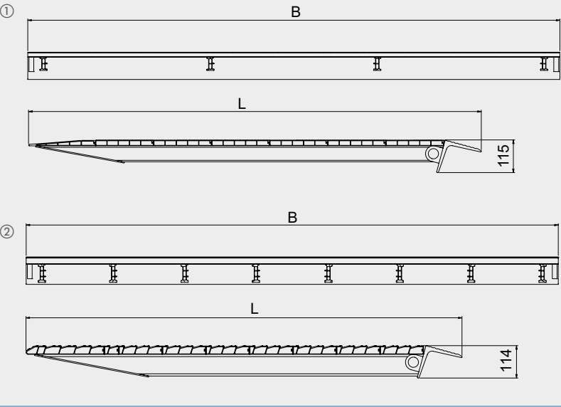
1 MODELLE SHL1 UND SHL2 2 MODELL SHL8
