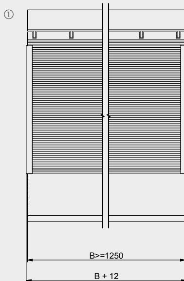
① MODELL MIT STAHSCHARNIEREN
